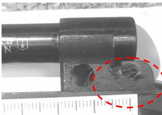
Рис. 11. Следы давления на штифте стойки ствола
