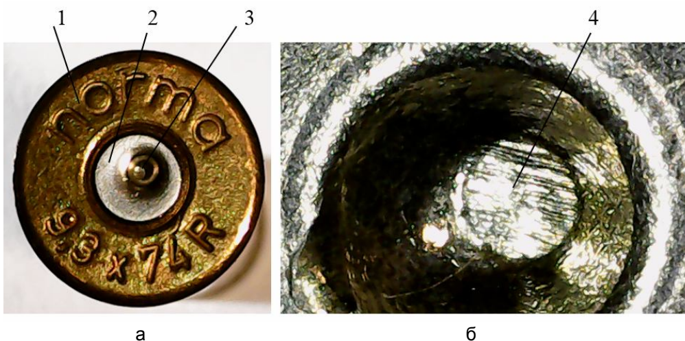
Рис. 2. Исследование следа бойка на капсюле стреляной гильзы: 1 – гильза; 2 – капсюль; 3 – след бойка; 4 – изображение на дне следа бойка
