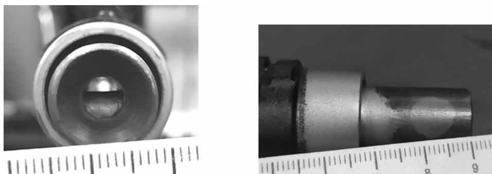
Рис. 1. Расположение штифта у дульного среза ствола (слева), вид шлифовки металла в месте расположения штифта сбоку от дульного среза ствола (справа)
