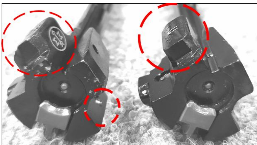
Рис. 3. Затвор: слева – автомата СХ-АК-12, справа – охотничьего карабина TR 3 калибра 5,45 × 39 мм
