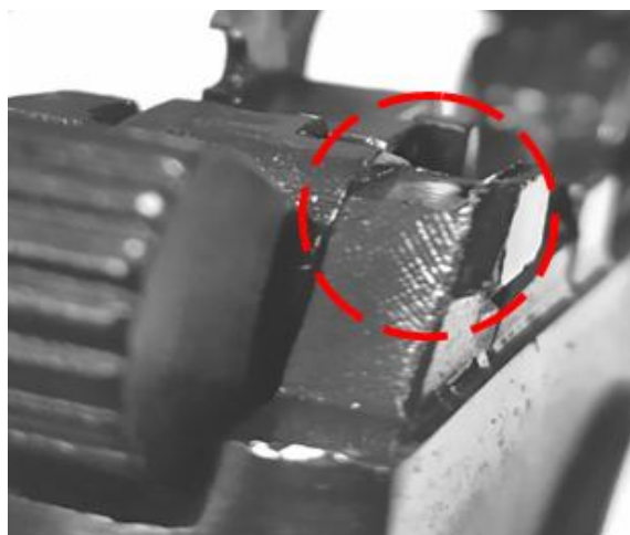
Рис. 12. Паз с правой стороны на рамке пистолета
