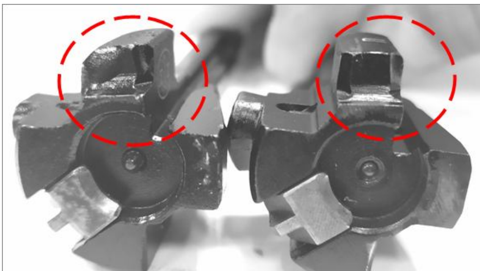
Рис. 6. Затвор: слева – автомата СХ-АК-103, справа – охотничьего карабина «Сайга МК» калибра 7,62 × 39 мм
