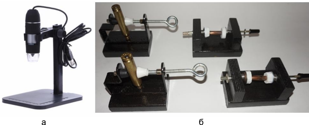
Рис. 1. Комплект для идентификационного исследования пуль и гильз: а – оптико-электронный микроскоп; б – держатели сравниваемых пуль и гильз
