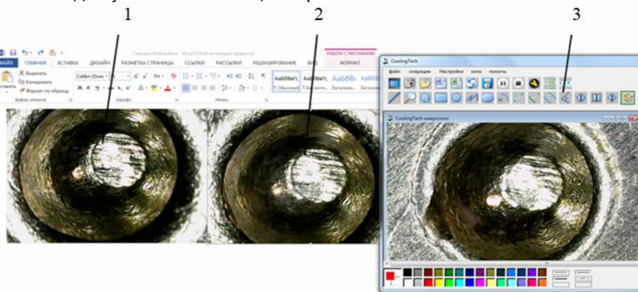
Рис. 3. Вывод изображений исследуемых следов бойка на монитор компьютера: 1 – гильза № 1; 2 – гильза № 2; 3 – подвижное окно микроскопа с изображением следа бойка
