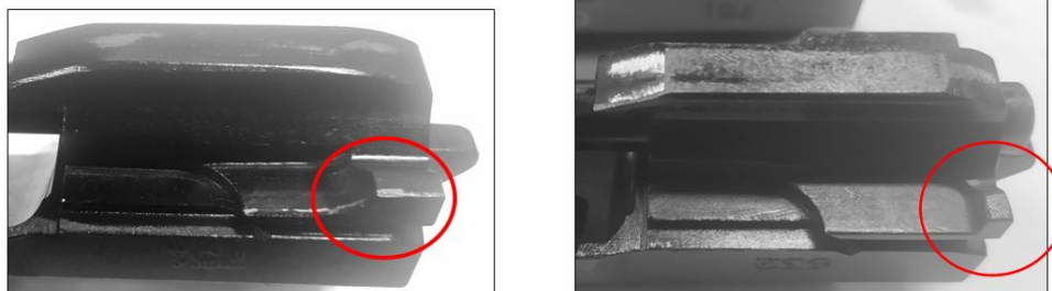
Рис. 7. Затворная рама: слева – автомата СХ-АК-103, справа – охотничьего карабина «Сайга МК» калибра 7,62 × 39 мм
